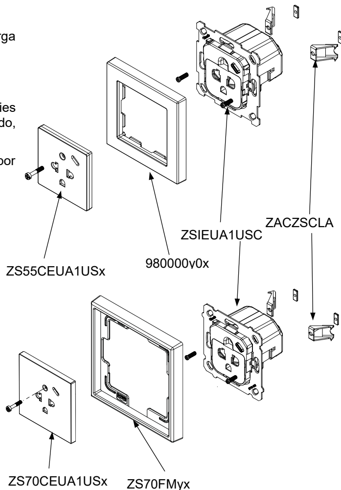
Figura 1. Base de enchufe euroamericano con USB tipo C
