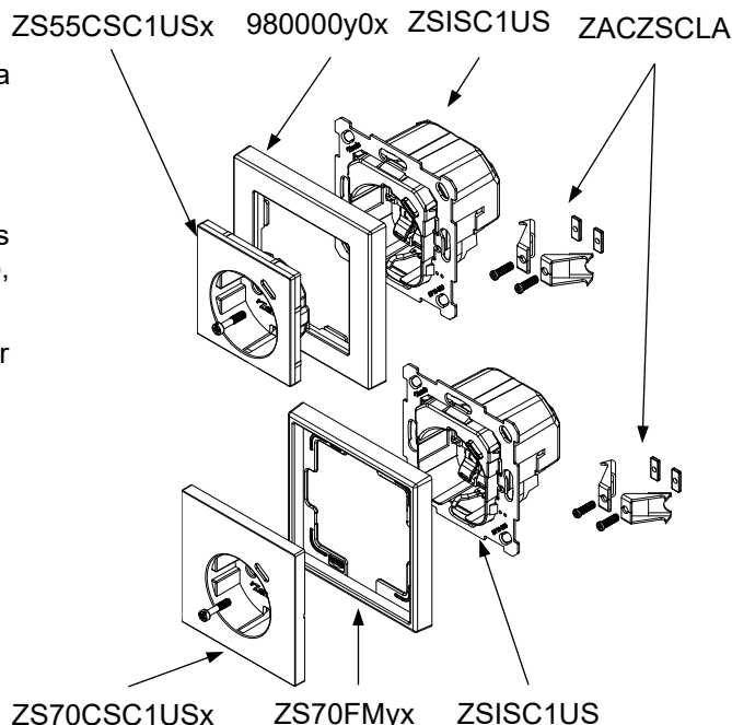
Figura 1. Base de enchufe Schuko con USB tipo C.
