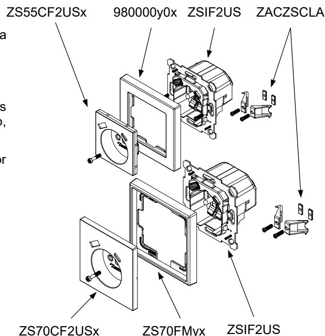
Figura 1. Base de enchufe francés con USB tipo A + C.
