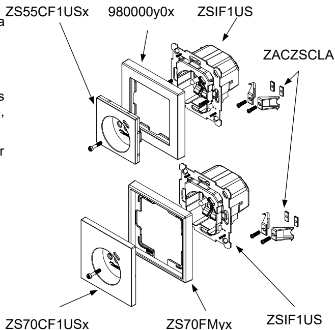
Figura 1. Base de enchufe francés con USB tipo C.
