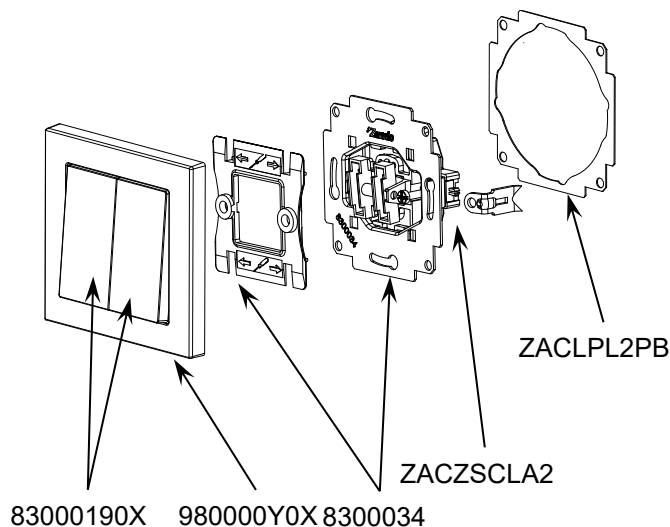
Figura 1. Conmutador doble
