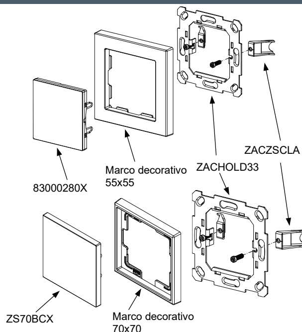
Figura 1. Tapa ciega.
