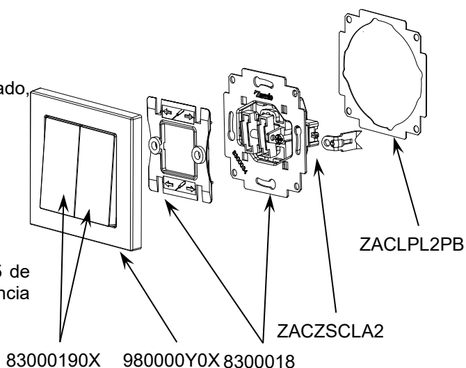
Figura 1. Interruptor doble
