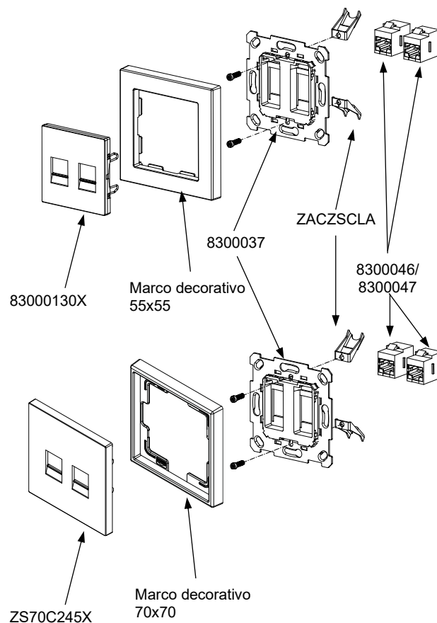
Figura 1. Toma RJ45 doble
