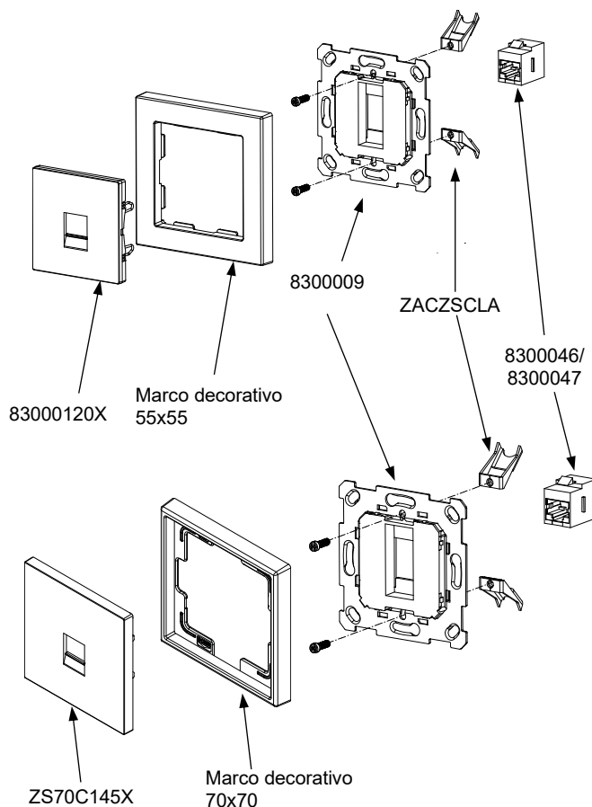
Figura 1. Toma RJ45 simple
