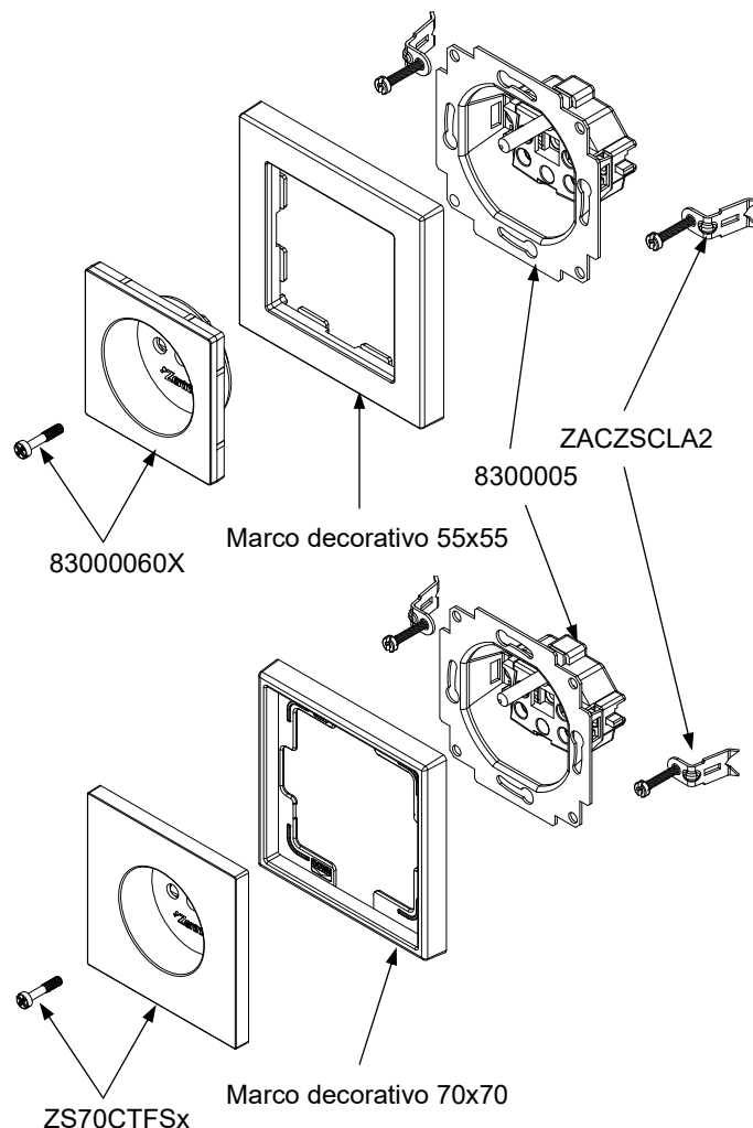
Figura 1. Toma de enchufe francés.
